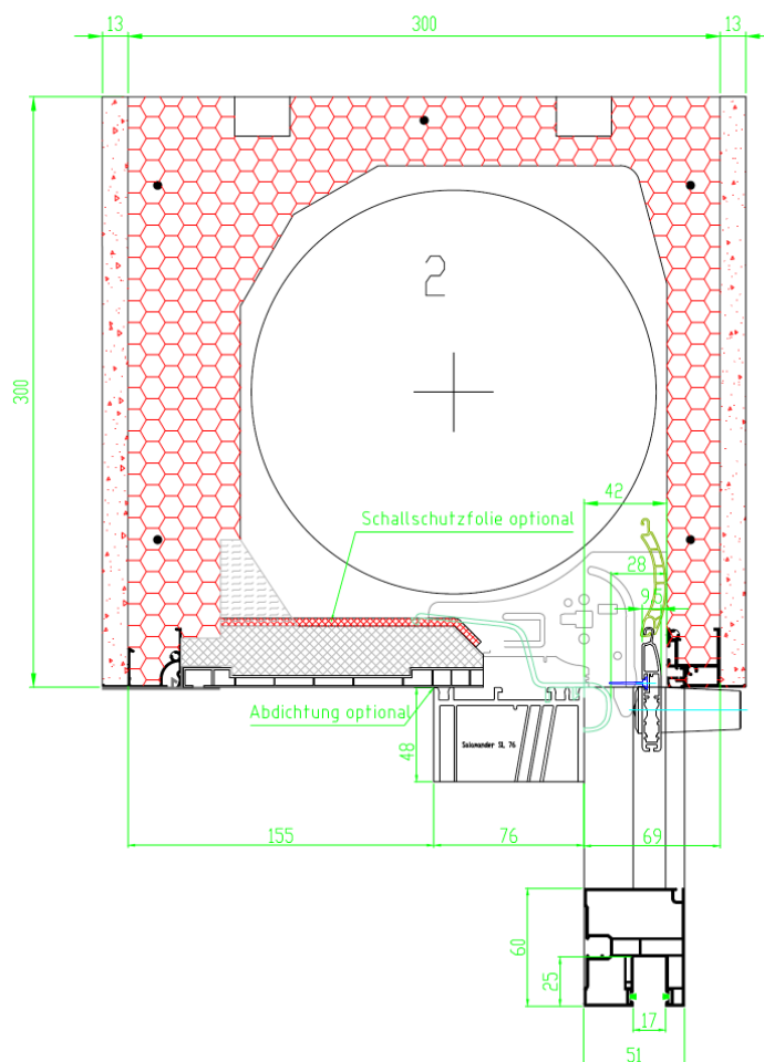
Bild 1 Schnittzeichnung (Grundsatzdetail, Ausführung ohne Schallschutzfolie, Anschluss an Fensterrahmen abgedichtet)
