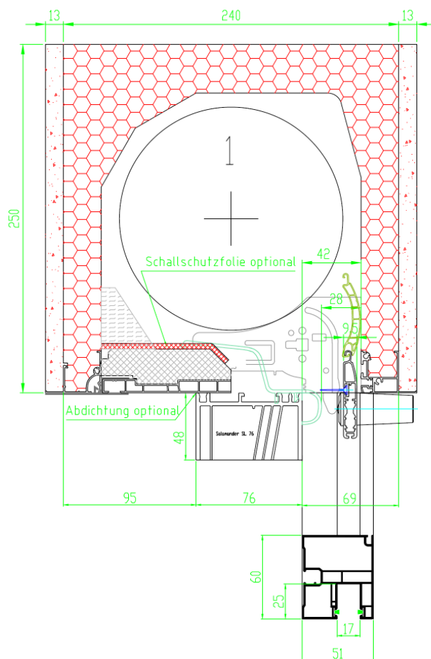
Bild 1 Schnittzeichnung (Grundsatzdetail, Ausführung mit Schallschutzfolie, ohne Abdichtung zum Fensterrahmen)
