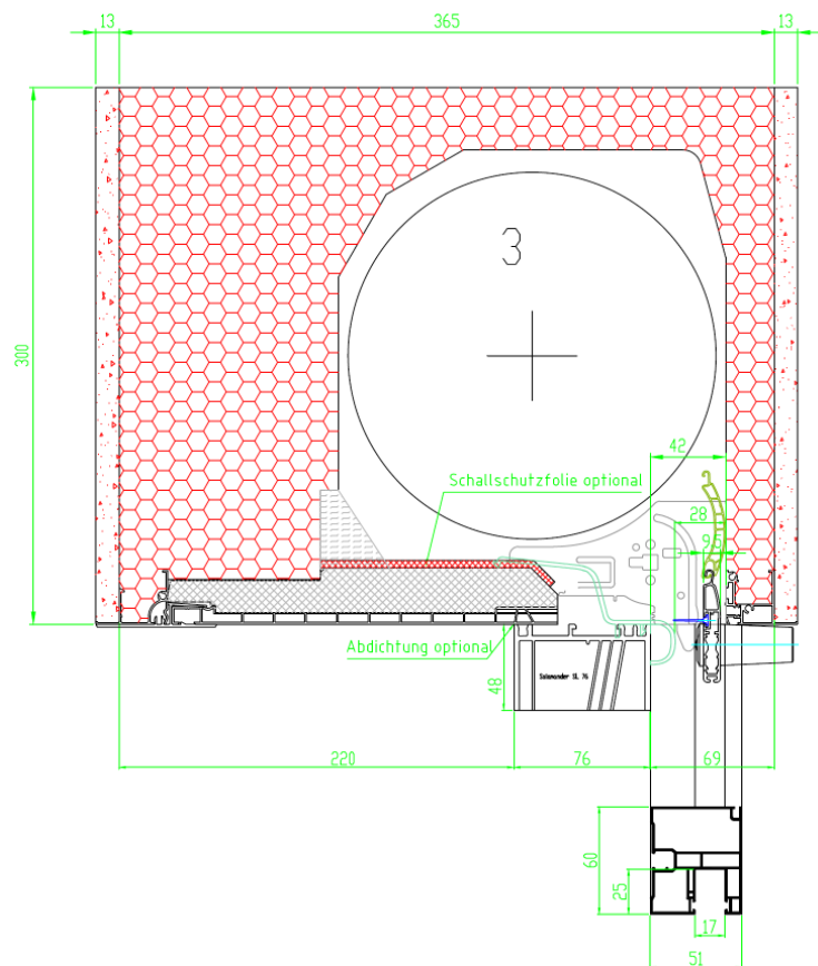
Bild 1 Schnittzeichnung (Grundsatzdetail, Ausführung mit Schallschutzfolie, Anschluss an Fensterrahmen abgedichtet)
