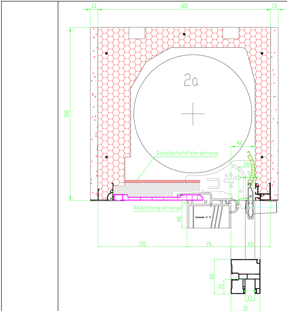
Abdichtung der Anschlussfuge zwischen Revisionsdeckel und Blendrahmen mit plastischem Dichtstoff, mit Schallschutzfolie
