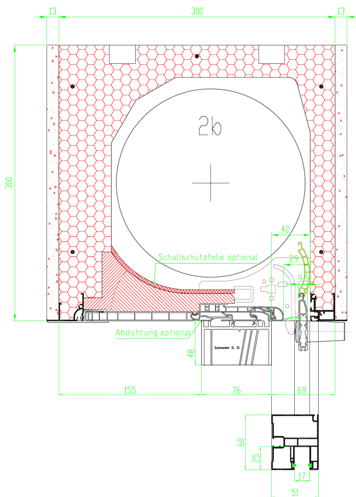
Bild 1 Schnittzeichnung (Grundsatzdetail, Ausführung ohne Schallschutzfolie und ohne Abdichtung zum Fensterrahmen)
