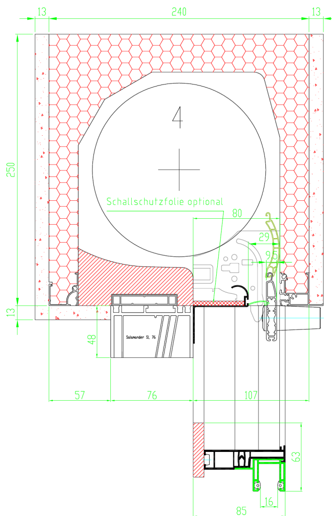
Bild 1 Schnittzeichnung (Grundsatzdetail, Ausführung ohne Schallschutzfolie)
